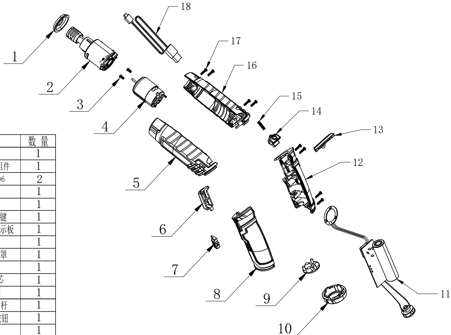
YSD401B螺丝批爆炸图
